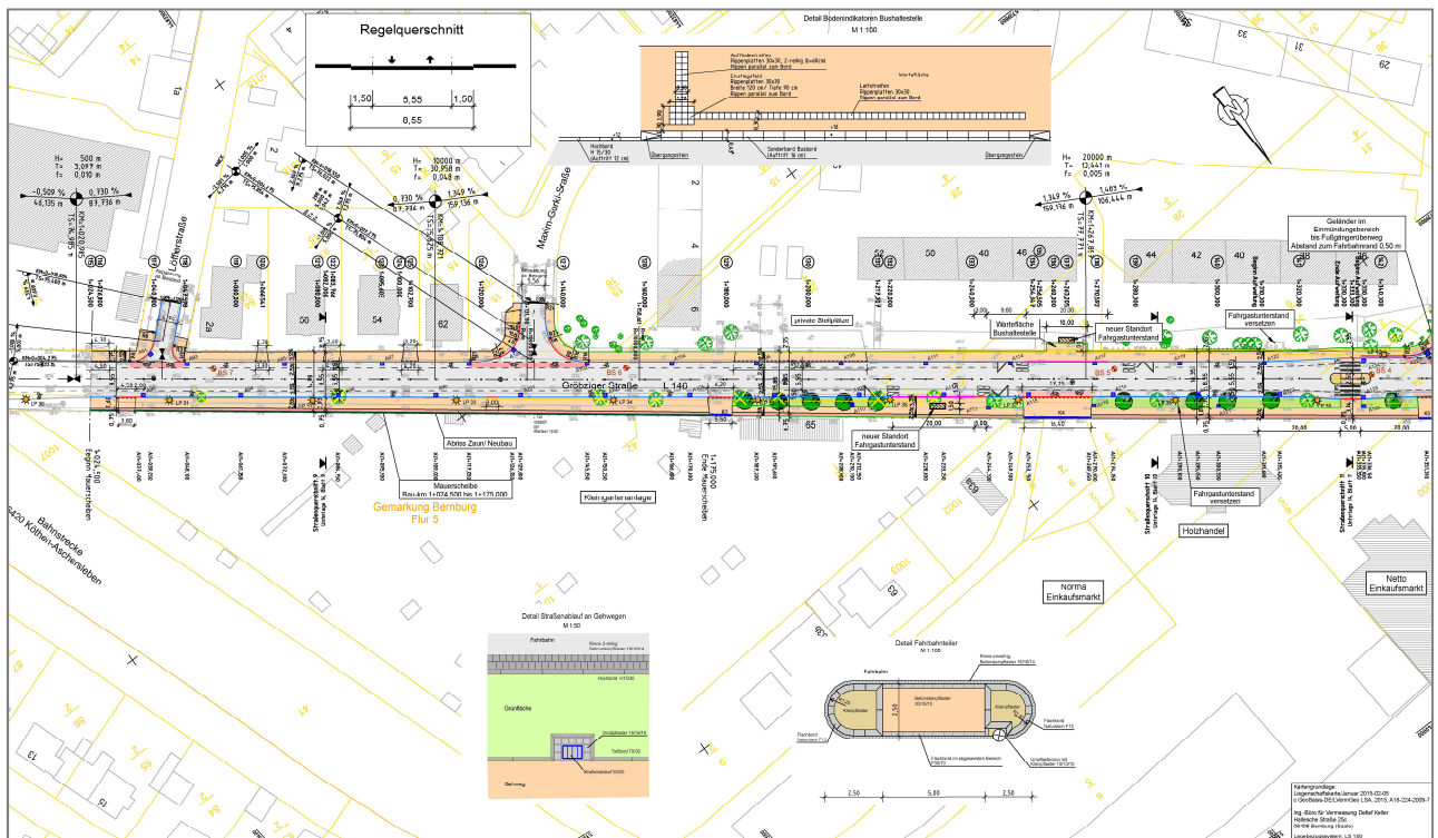
Abbildung 2: Landesstraßenbaubehörde Sachsen-Anhalt, Regionalbereich West, Lageplan zum grundhaften Ausbau der L 146 OD Bernburg Gröbzigter Straße/Thomas-Müntzer-Straße in Bernburg (Saale) – Ausführungsplanung, Planungsbüro: Baumeister Ingenieurbüro GmbH Bernburg
