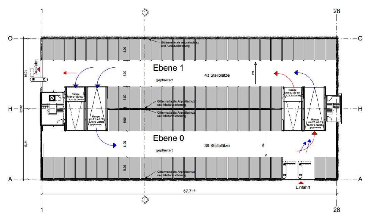
Grundriss Ebenen 0 und 1
