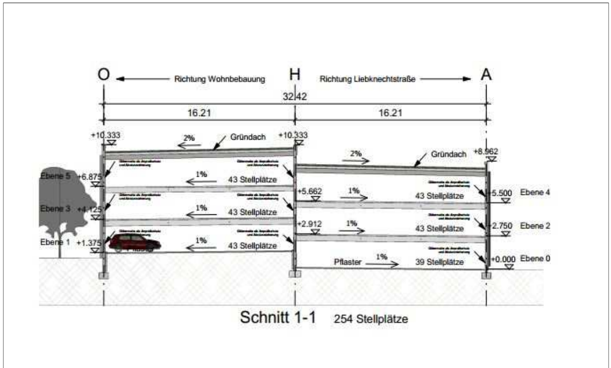
Schnitt 1 - 1
